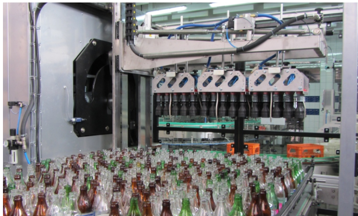
Bottle unloader NAPAK 3 PIWNICZANKA ZBNWM Sp.P., Poland
